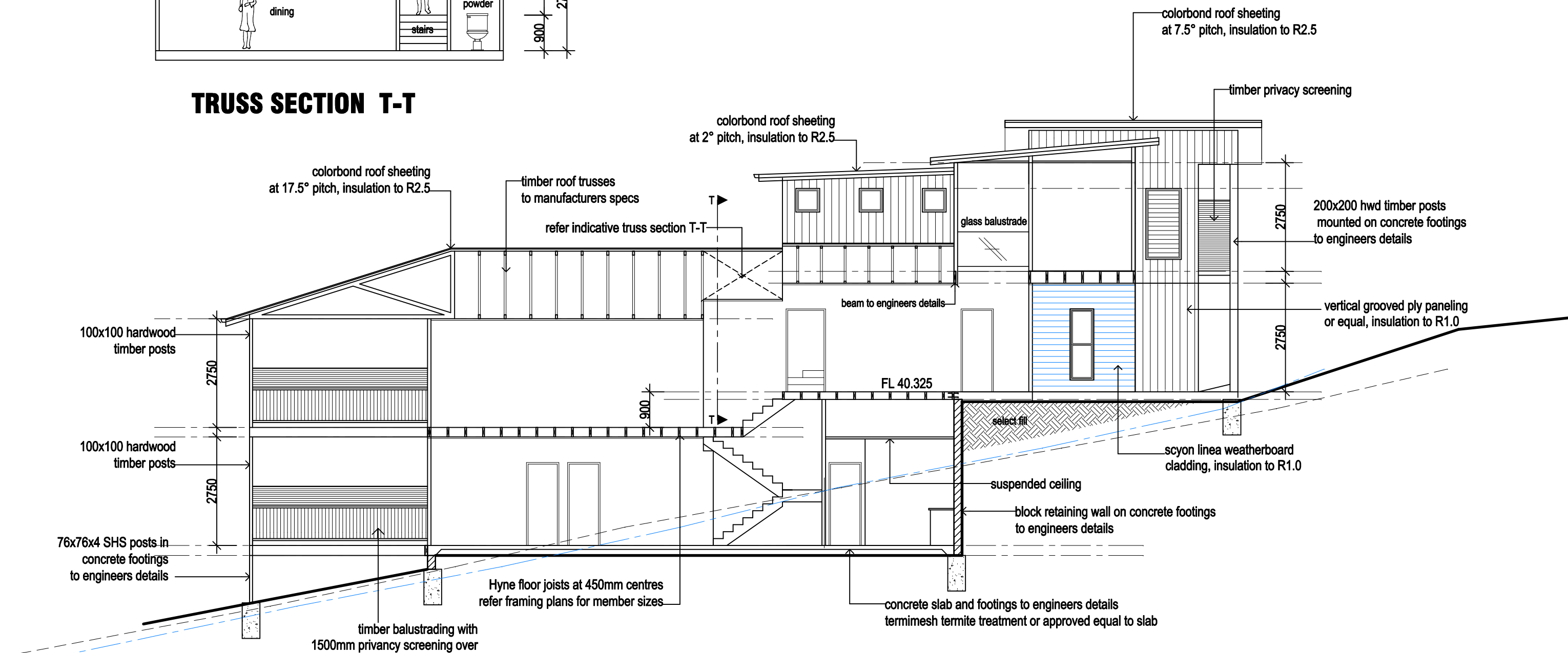
SECTION A-A
